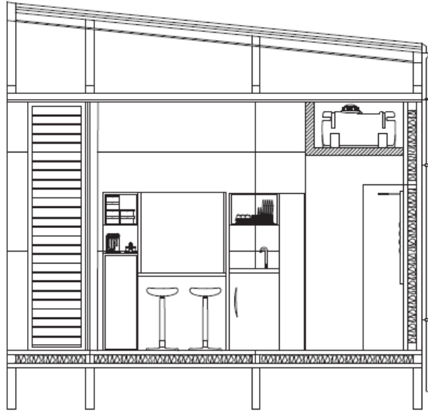
CORTE A-A
