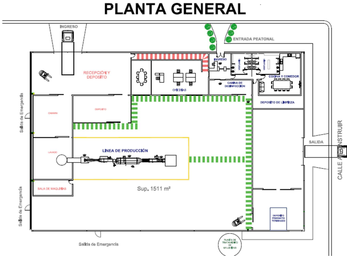
Gráfico XII: Plano de distribución de las áreas de la planta.
